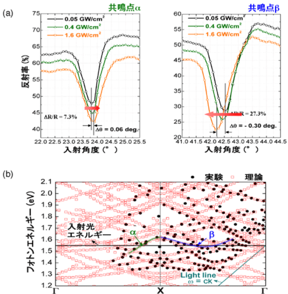
図2 (a) 角度分解反射スペクトルの入射光強度依存性。共振点 a、b はそれぞれ異なる光バンドに共振した状態であり、共振点 b において大きな非線形変化が生じていることが分かる。
