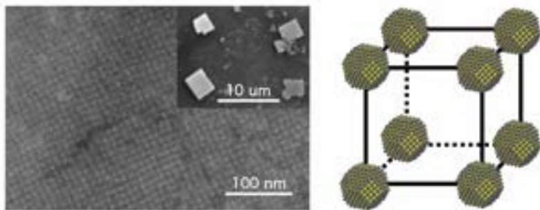
PbS コロイド量子ドットが単純立方格子状に集合した超結晶、その超結晶表面の電子顕微鏡像、充填様式図
