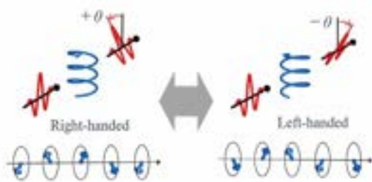
らせんスピンがつくる自然旋光性とその制御
