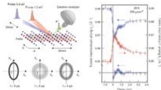
時間分解角度分解光電子分光 (左上)、フェルミ面過渡応答の模式図 (左下) および得られたフェルミ波数の超高速時間変化 (右)
