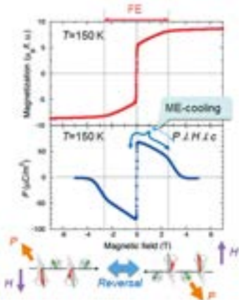
Y型六方晶フェライト BaSrCo 2 Fe 11 AlO 22 における磁場誘起電気分極反転と磁気秩序の変化
