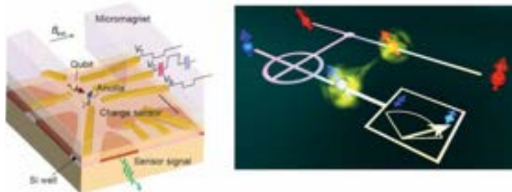
図(左) 実験に用いた二重量子ドット試料の模式図。(右) 量子非破壊測定の概念図。
