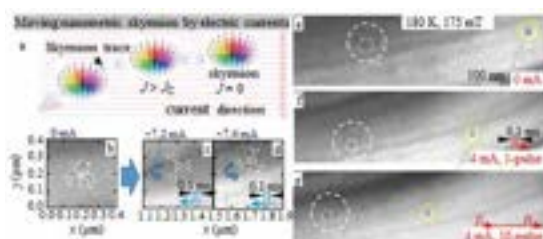
(a) 電流下のスキルミオンホール運動の模式図。 (b-d) 電流パルス印加前 (b) と印加後 (c-d) のスキルミオンクラスタの回転運動のローレンツ電子顕微鏡像。(e-g) 電流パルス印加前 (e) と印加後 (f-g) のローレンツ電子顕微鏡像。
