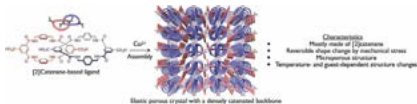
カテナンからできた柔軟な多孔性結晶
