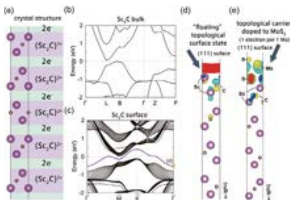
(a) トポロジカル電子化物 [Sc_2C]^{2+}2e^- の結晶構造, (b) Sc_2C のバンド構造, (c) Sc_2C (111) 表面のバンド構造, (d) 宙に浮かんだトポロジカル表面状態, (e) MoS_2 に注入されたトポロジカル電荷
