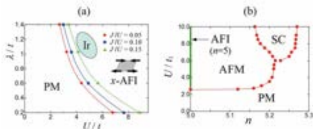
スピン軌道相互作用を取り入れた3軌道ハバード模型の基底状態相図 (a) 電子密度 n=5 、(b) n>5
