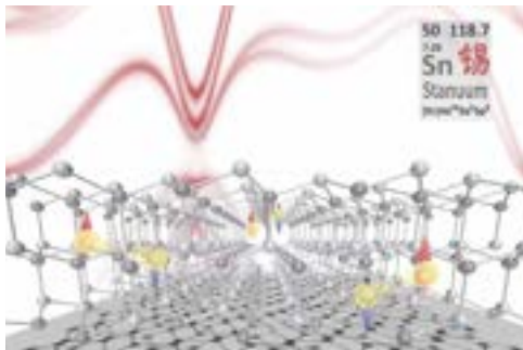
スタネンの結晶構造とイジング的クーパー対の概念図。 赤線はバンド分散であり、右上には錫の情報を示す。
