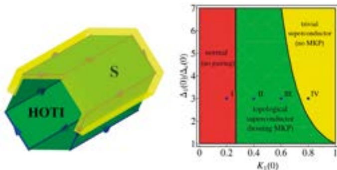
左図：超伝導体(黄色)と細線(緑)による高次トポロジカル絶縁体の概念図
