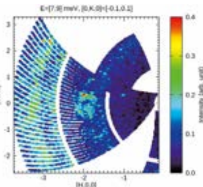
(H 0 L)に観測された格子励起スペクトラム (T=300K, 7<E<9 meV)
