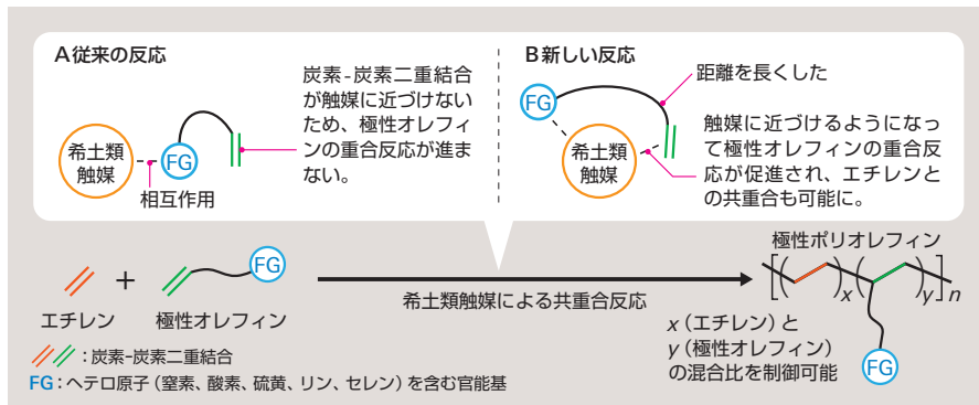
図3 希土類触媒によるエチレンと極性オレフィンとの共重合反応
