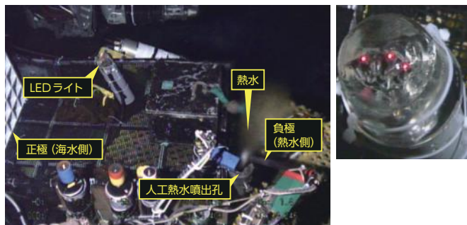
図2 人工熱水噴出孔における熱水—海水燃料電池の発電実験 左は熱水—海水燃料電池の全体写真。熱水側と海水側に電極を設置して電線をつなぎ、その間にLEDライトを入れてある。右は3個の赤色のLEDが点灯した様子。人工熱水噴出孔とは、海底下の熱水だまりから海底面までパイプを通し、パイプの先端から熱水が噴き出すようにしたもの。(提供:海洋研究開発機構)
