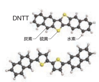
図3 DNTT(ジナフトチエノチオフェン)と一般的なp型有機半導体(下)の構造
