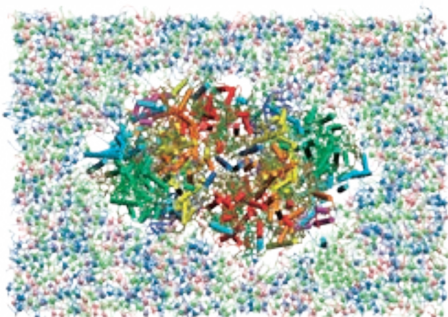
光合成膜タンパク質PS II
